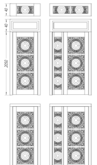
Модель 303 Тільки 16 мм МДФ
