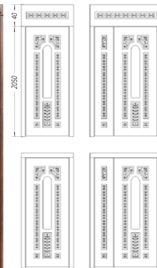
Модель 318 Тільки 16 мм МДФ
