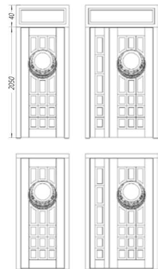
Модель 308 Тільки 16 мм МДФ
