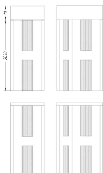
Модель 417 Тільки 16 мм МДФ
