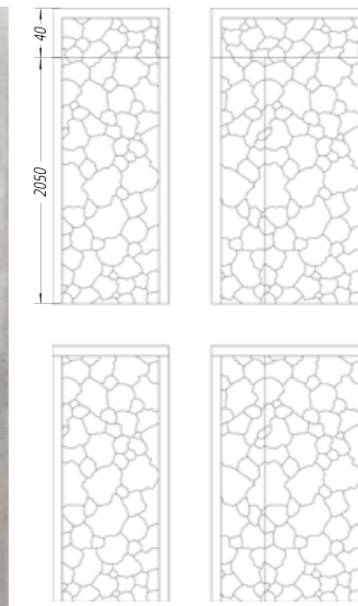
Модель 419 Тільки 16 мм МДФ
