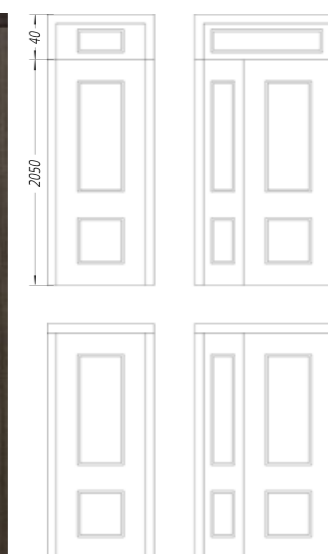
Модель 421 Тільки 16 мм МДФ
