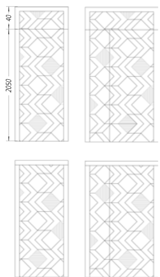
Модель 80 Тільки 16 мм МДФ
